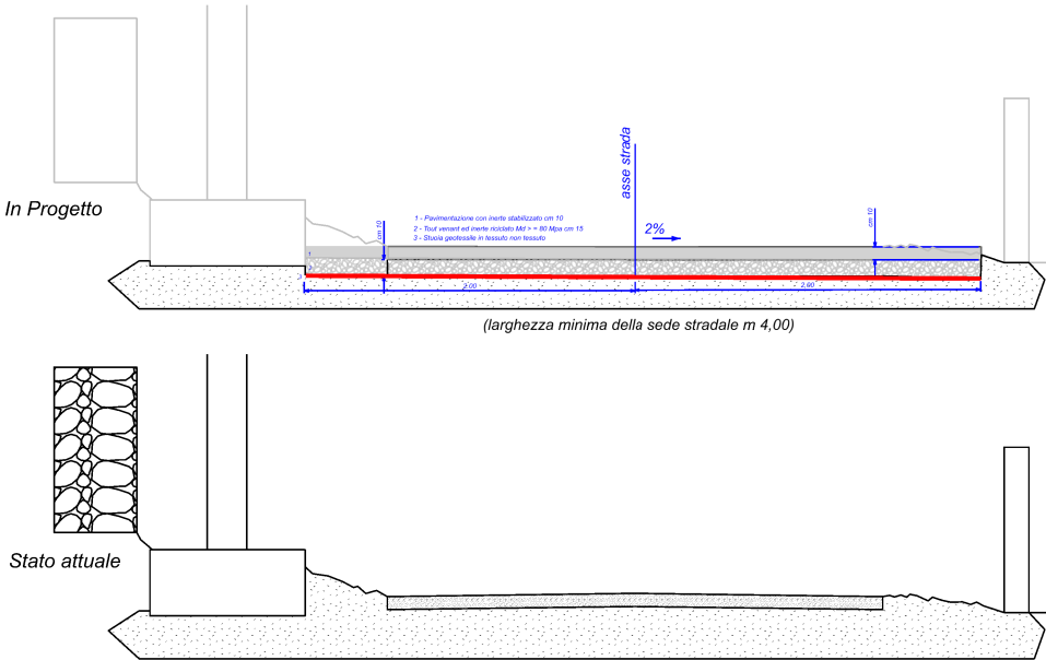
Sezione Tipo segmento 2 "in forte pendenza"
