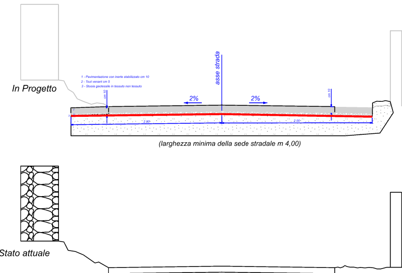
Sezione Tipo segmento 3 "a monte"
