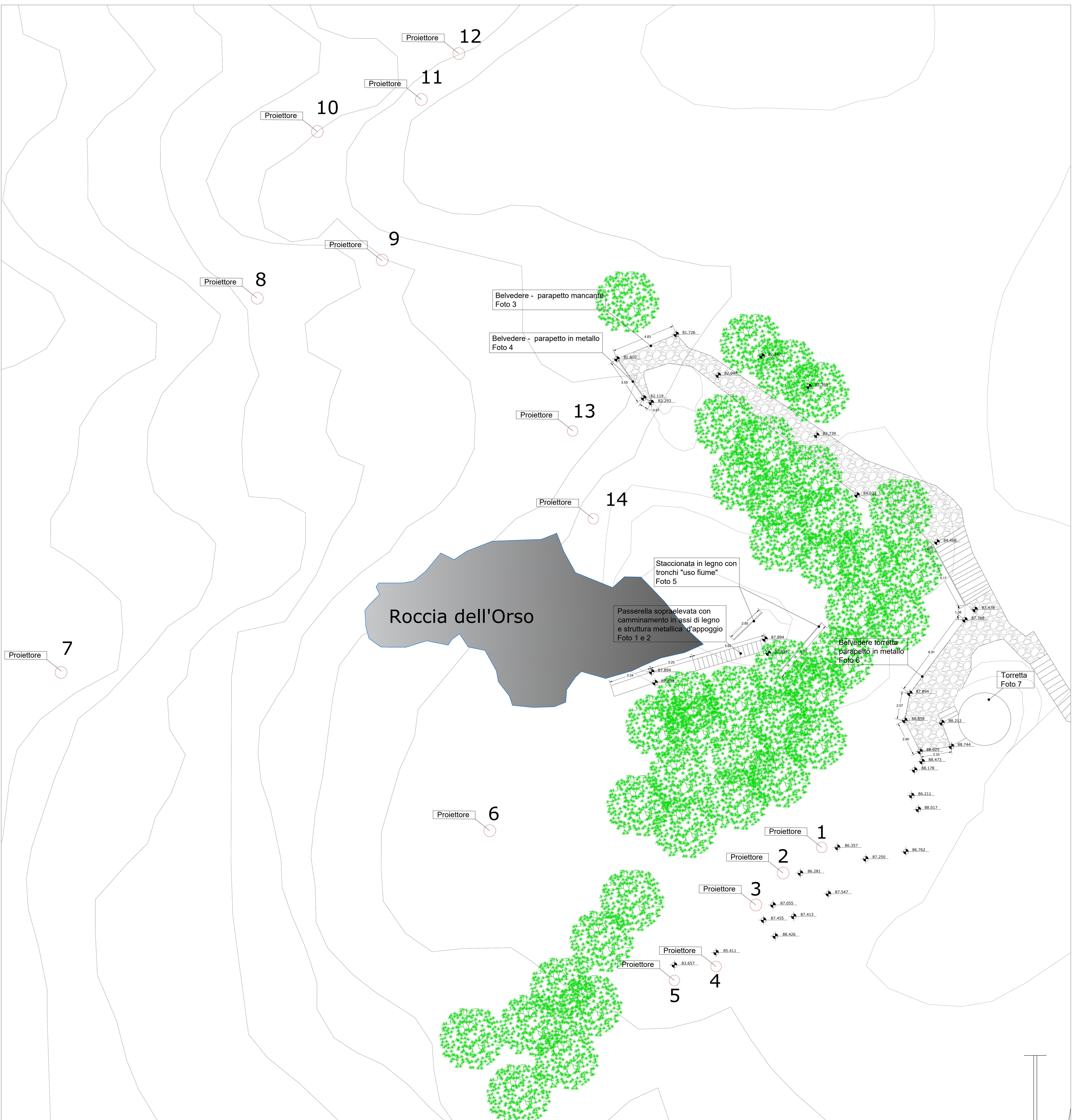
Planimetria piano quotato CTR scala 1:100
