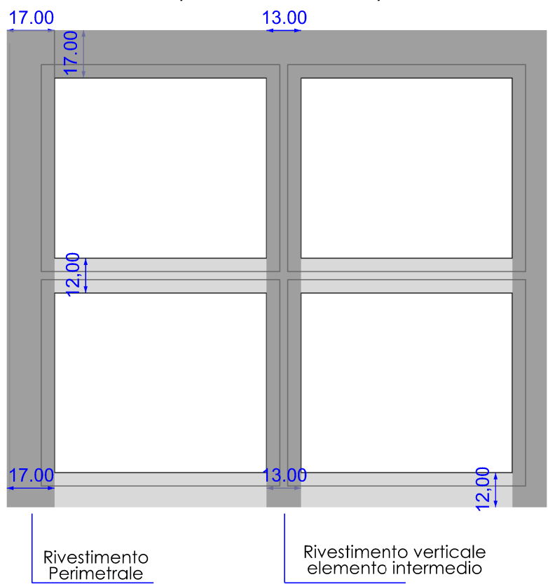
Particolare cornici di rivestimento in granito (dimensioni in cm)
