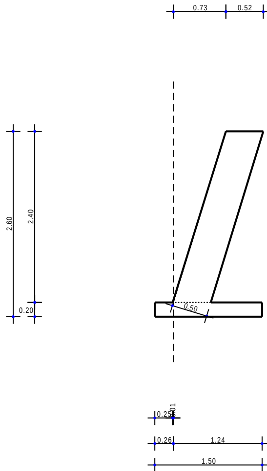
Sezione... - Vista Sezione
