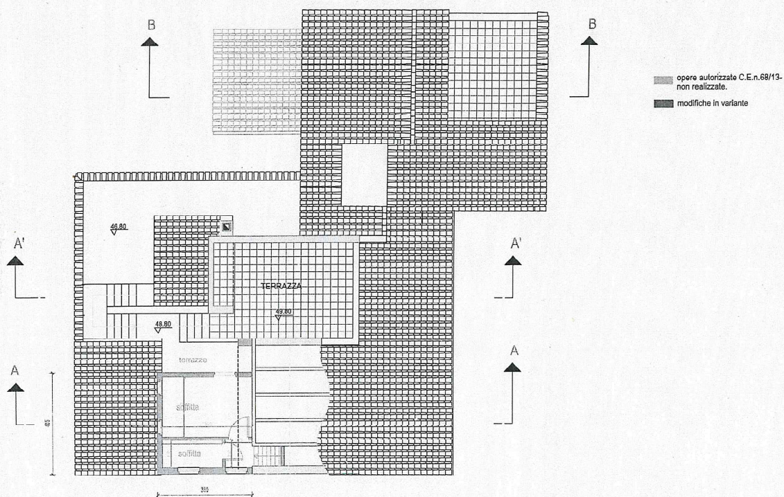
Modifiche in Variante PIANO SOFFITTA E TERRAZZA-1:100
