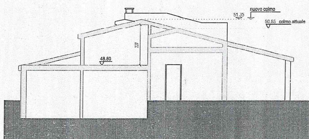
Stato Autorizzato SEZIONE A - A - 1/100
