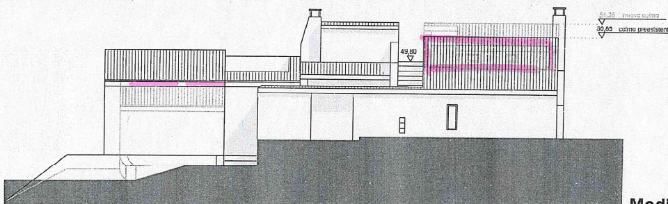
Modifiche in variante PROSPETTO SUD-OVEST-1/100
