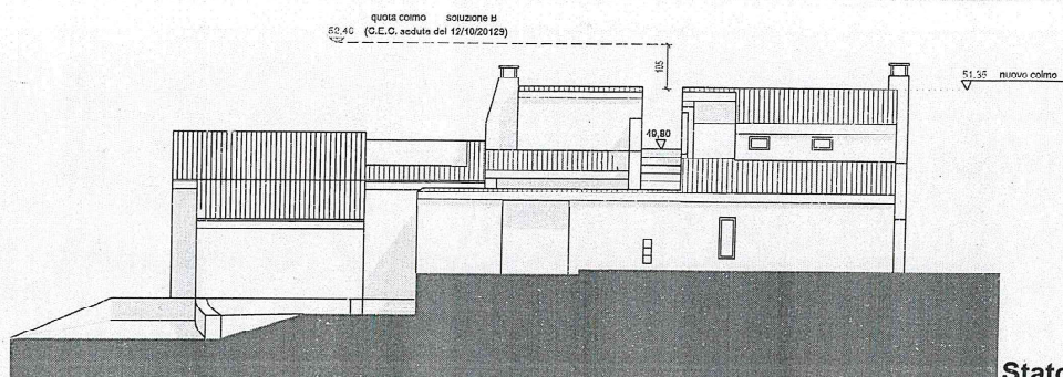
Stato Autorizzato PROSPETTO SUD-OVEST-1/100
