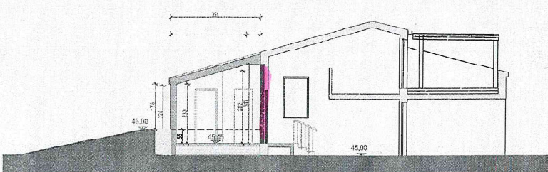
Modifiche in variante SEZIONE A - A - 1/100
