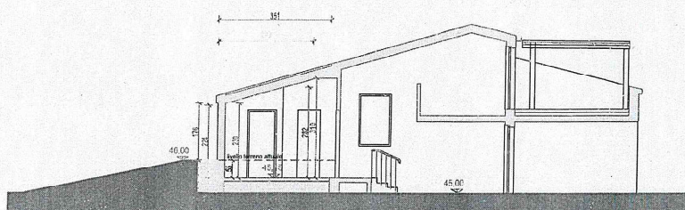
Stato Autorizzato SEZIONE A - A - 1/100
