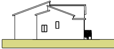
PROSPETTO NORD IN PROGETTO
