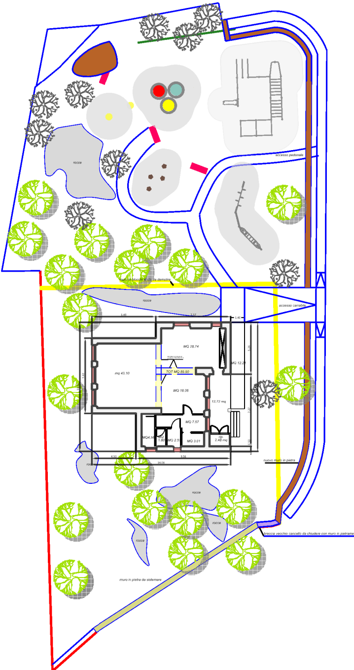
PIANTA QUOTATA IN PROGETTO 1:100
