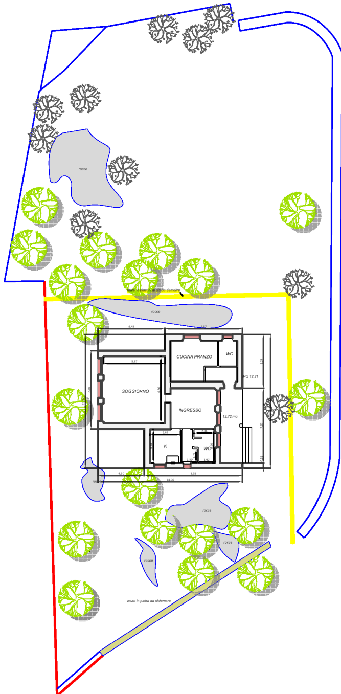
PIANTA QUOTATA ESISTENTE 1:100
