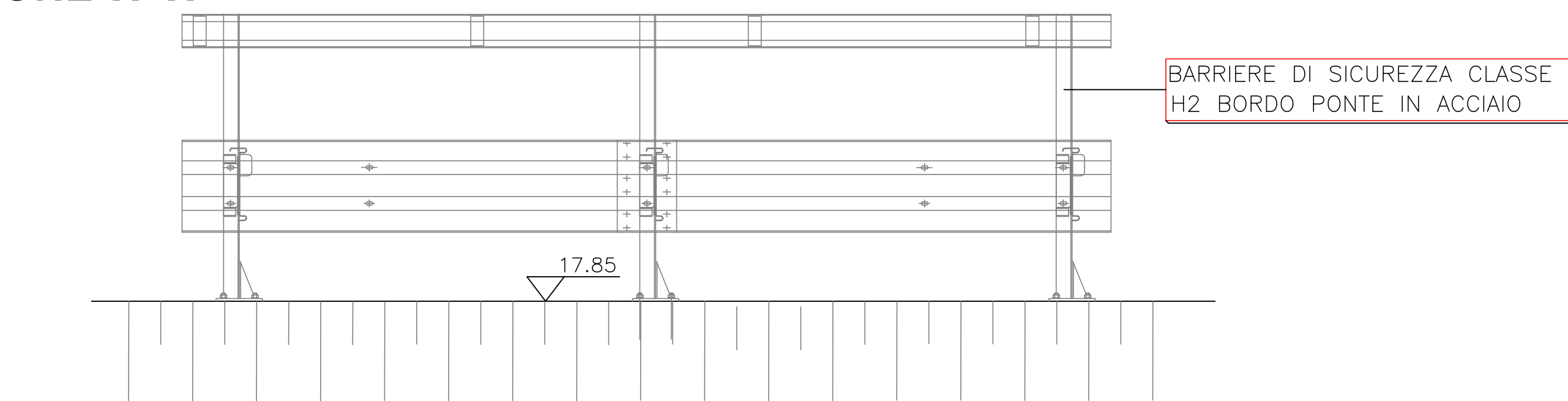
SEZIONE W-W'
