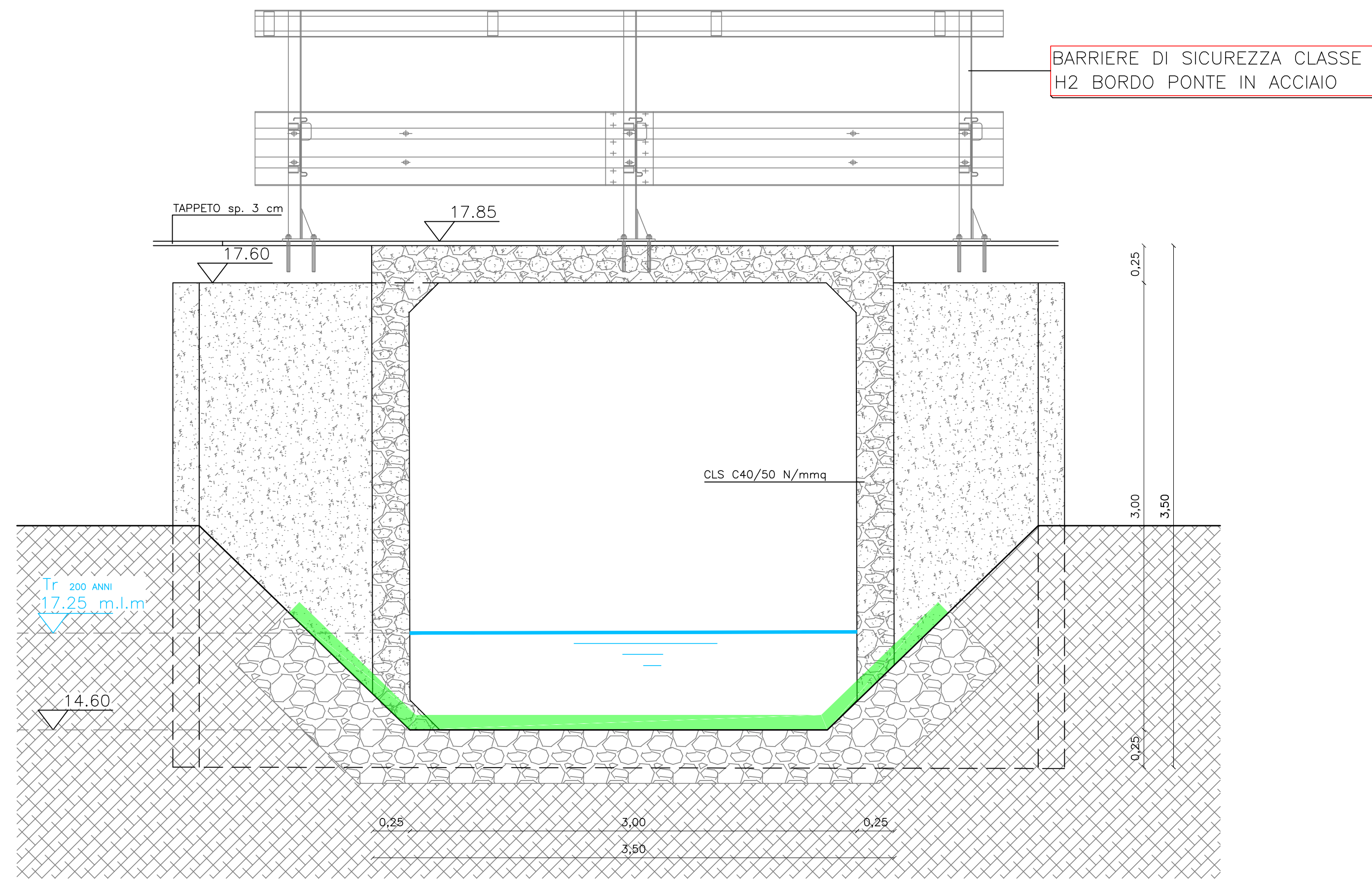
SEZIONE W-W'
