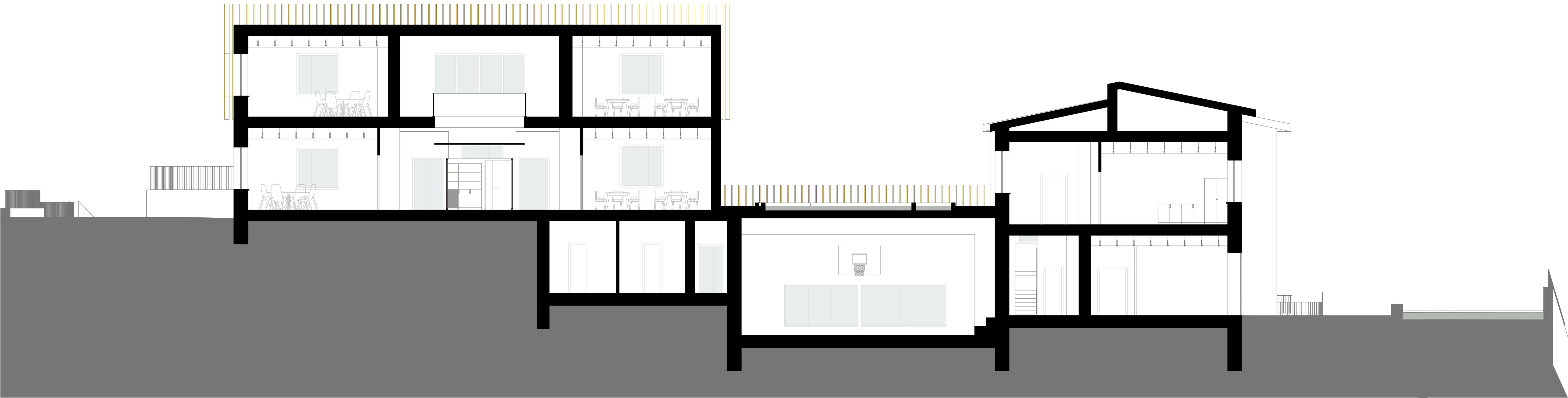
Sezione BB |
