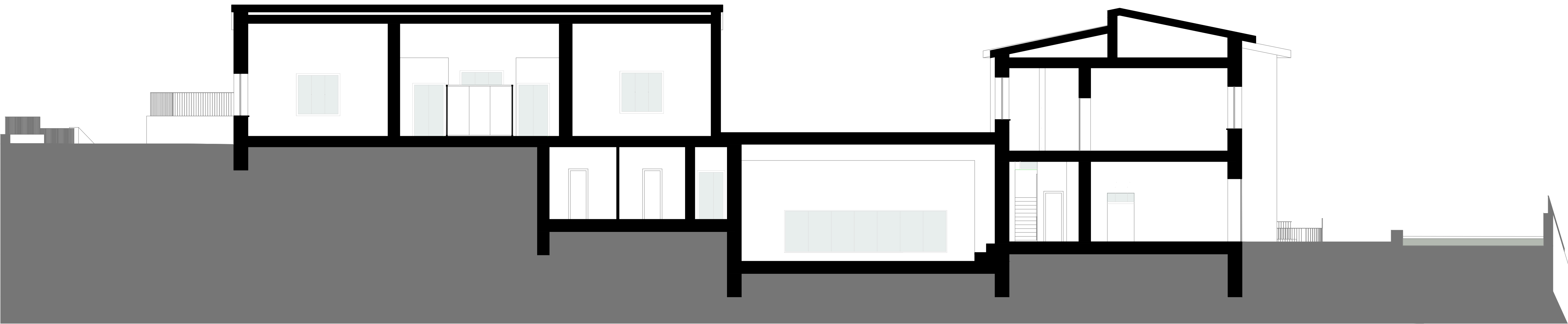
Sezione BB |
