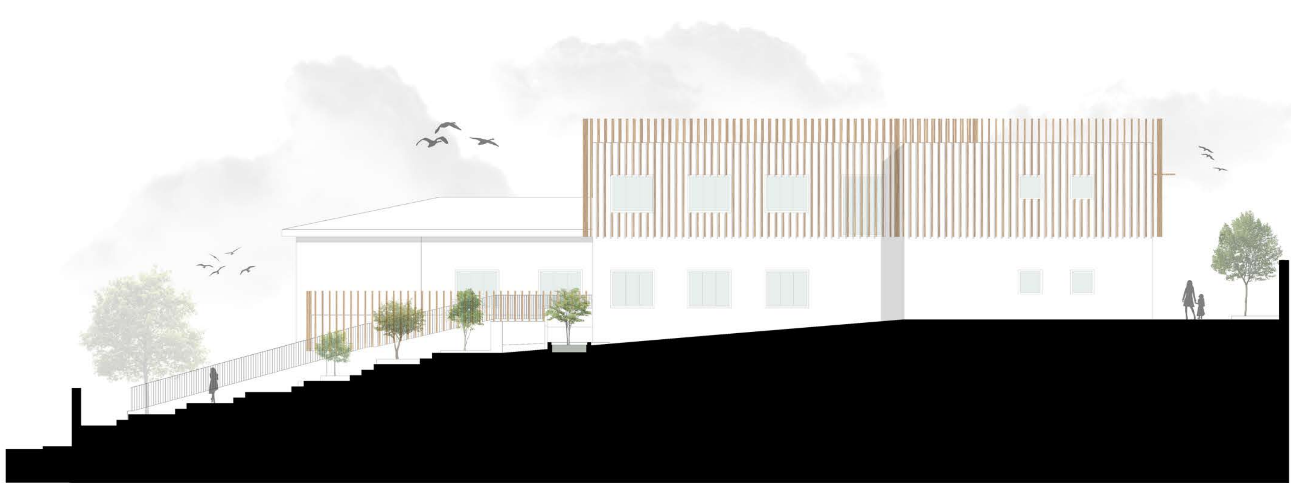
PROSPETTO OVEST
