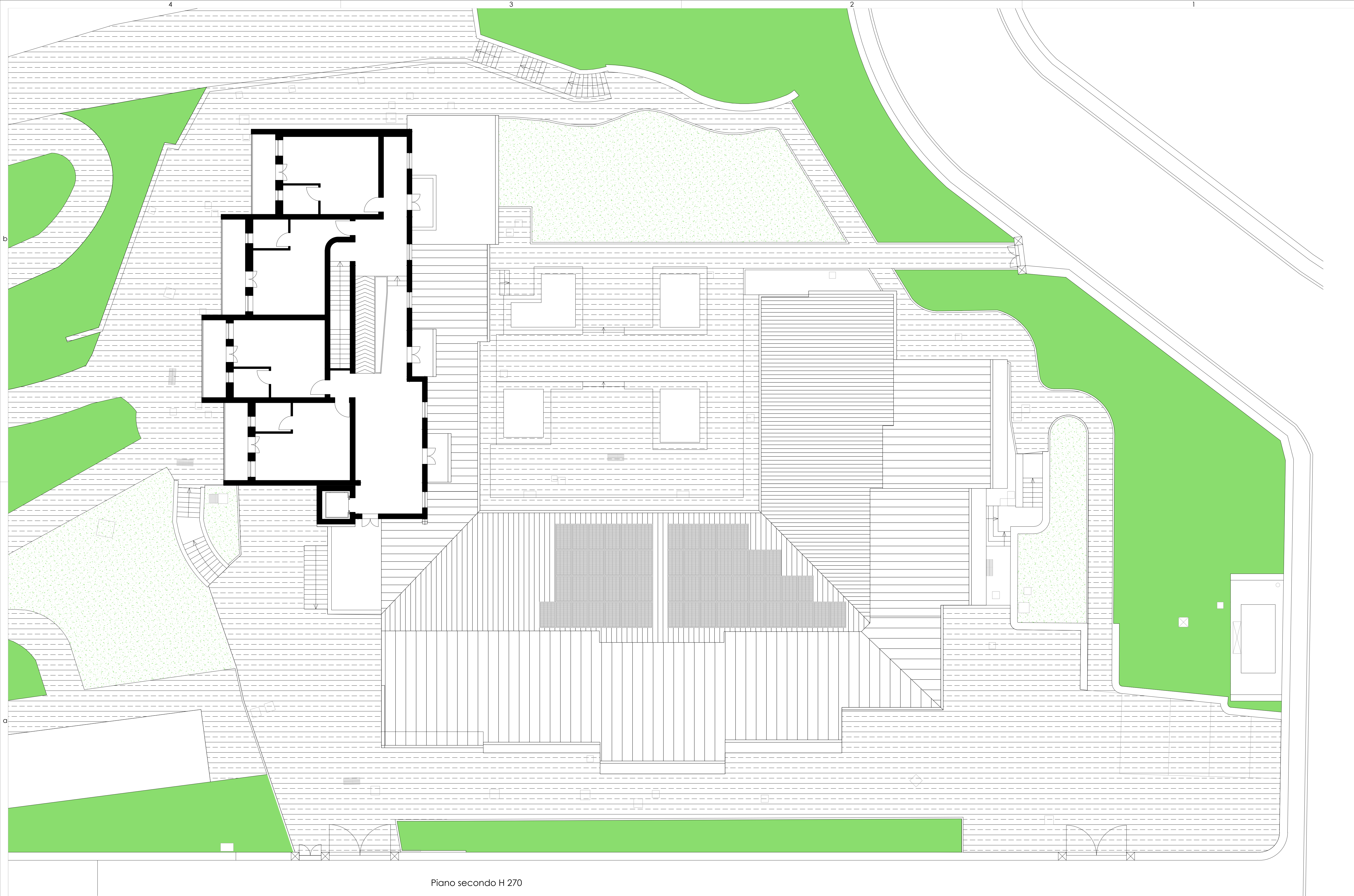
PLANIMETRIA PIANO SECONDO - stato di fatto Scala 1:100
