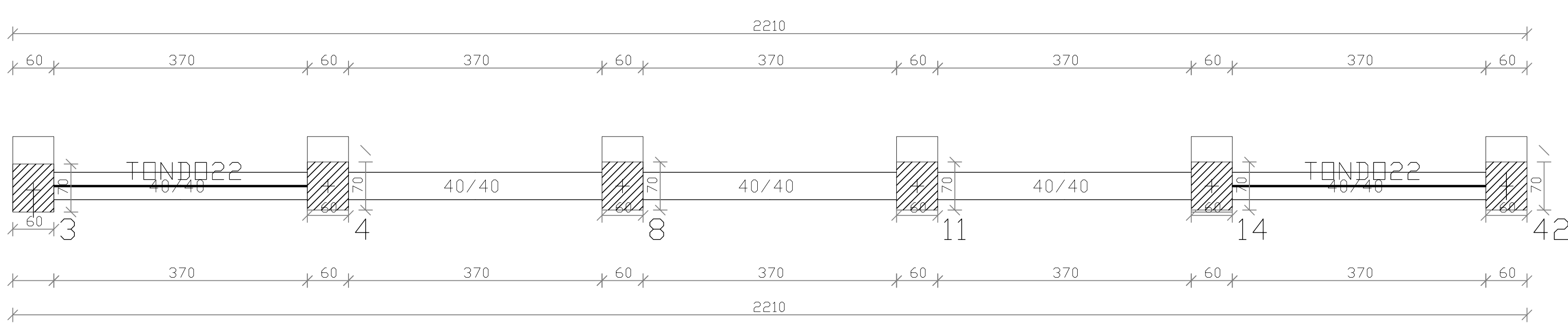
PIANTA IMPALCATO QUOTA m: 6.65
