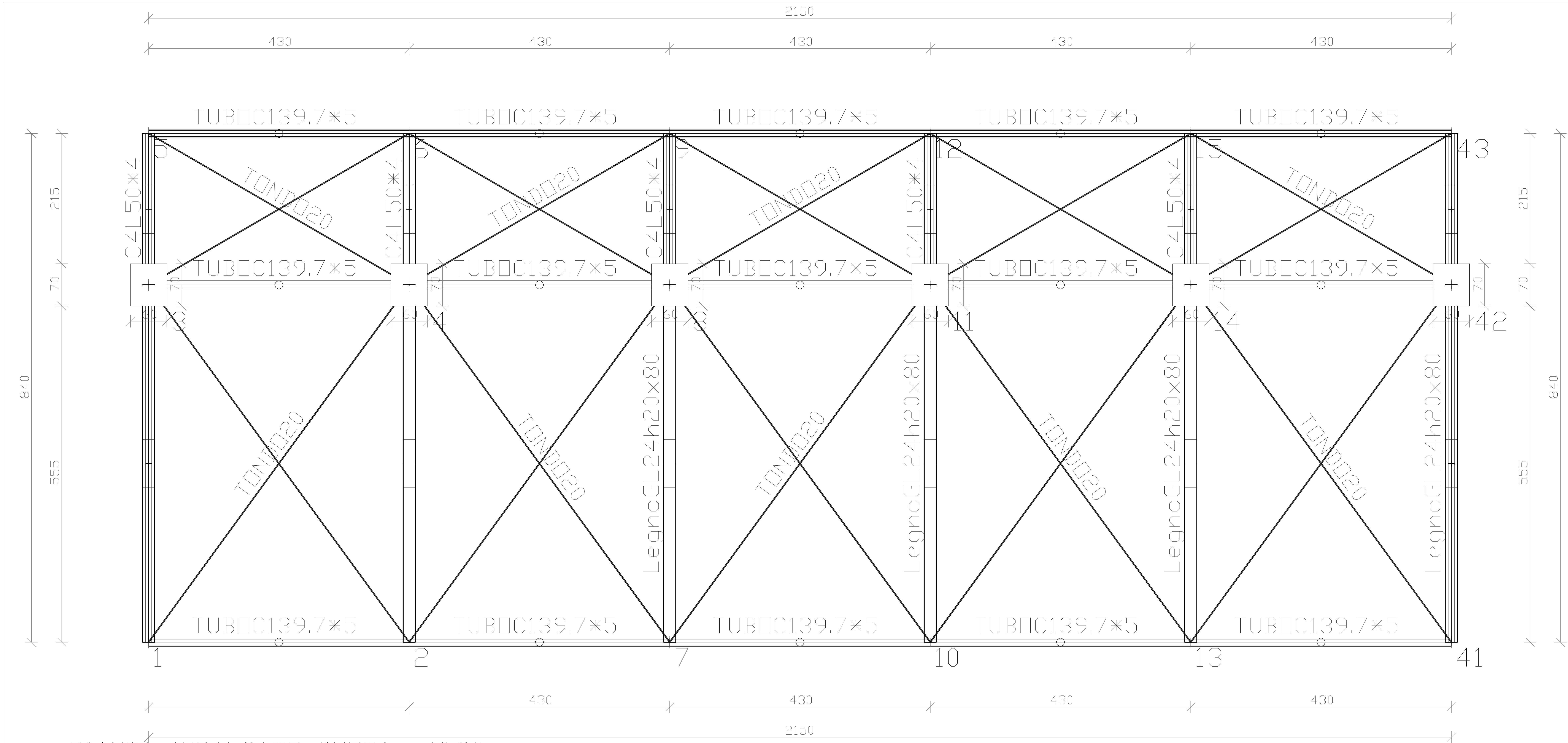
PIANTA IMPALCATO QUOTA m:10.30
