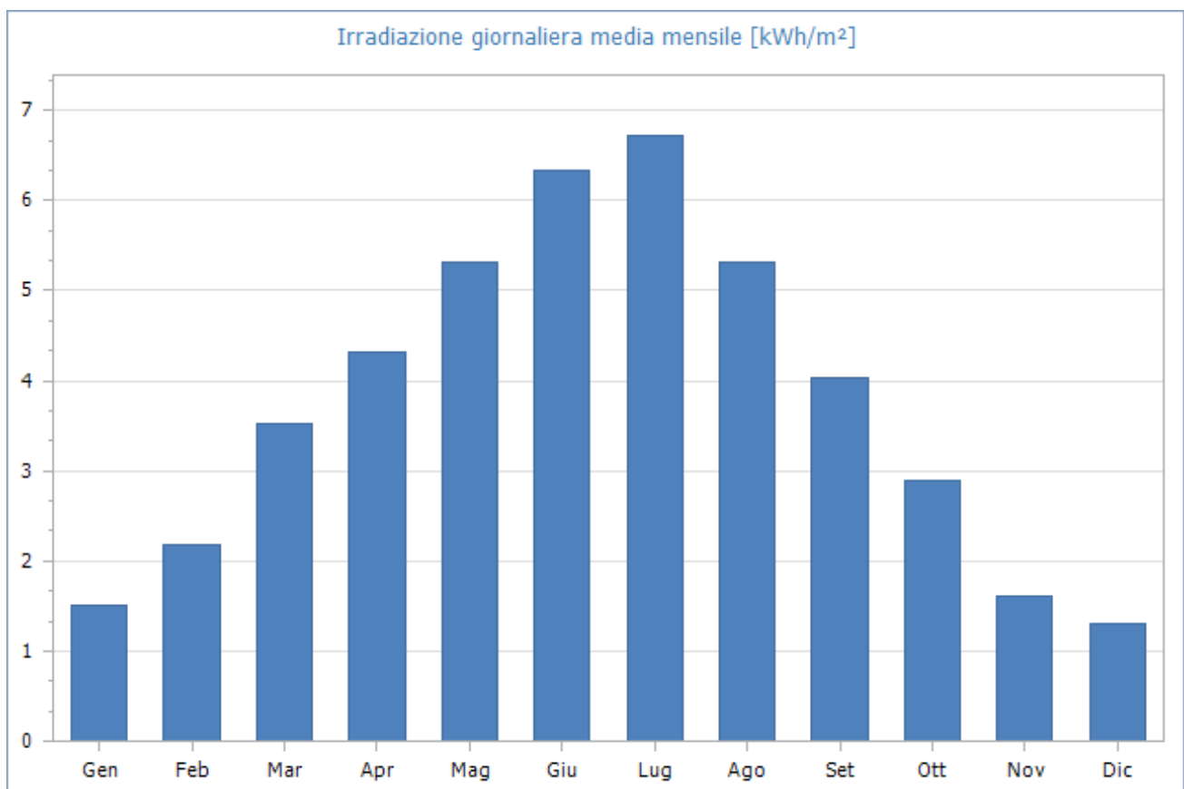
Fig. 1: Irradiazione giornaliera media mensile sul piano orizzontale [kWh/m 2 ]- Fonte dati: UNI 10349:2016 - Stazione di rilevazione: Luras
