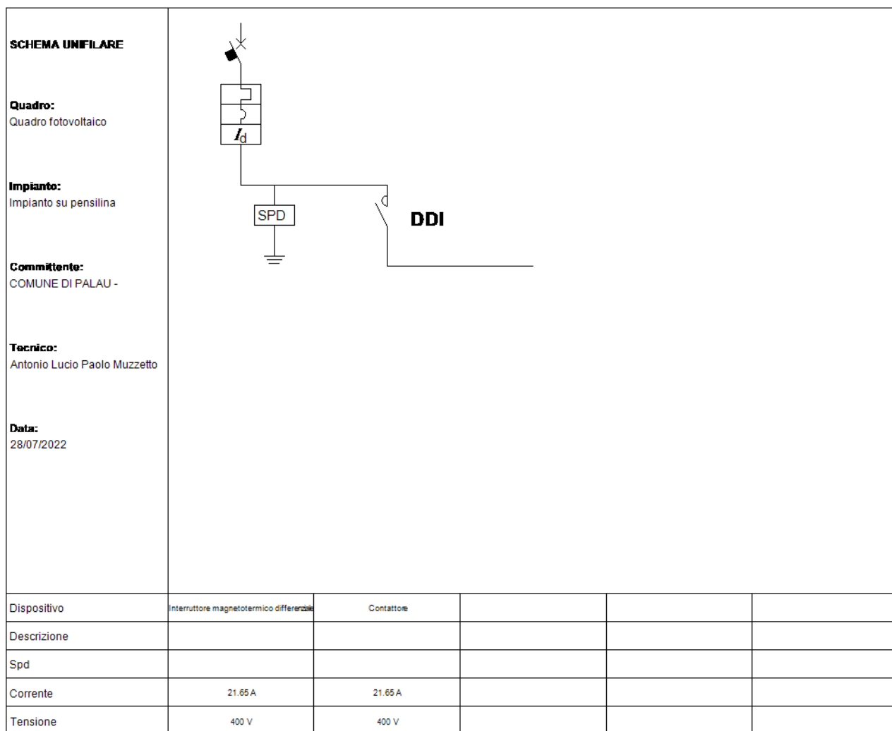
Fig. 5: Schema unifilare quadro "Quadro fotovoltaico"
