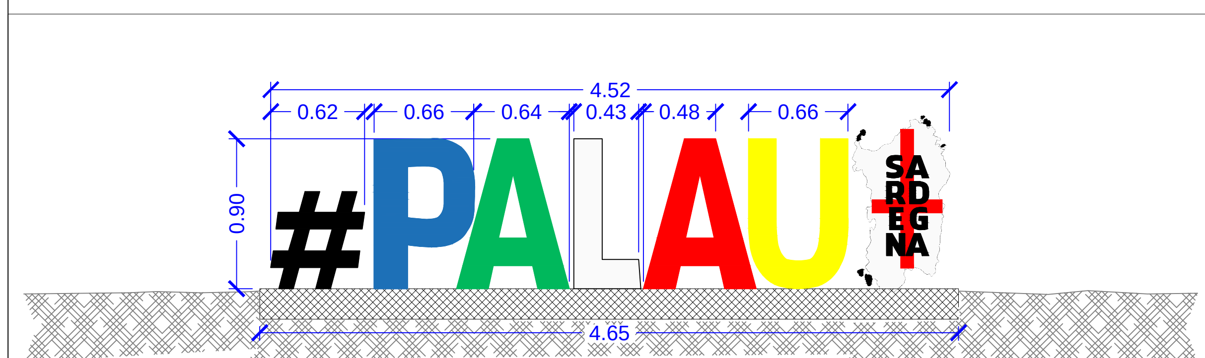
Prospetto Insegna scala 1: 25
