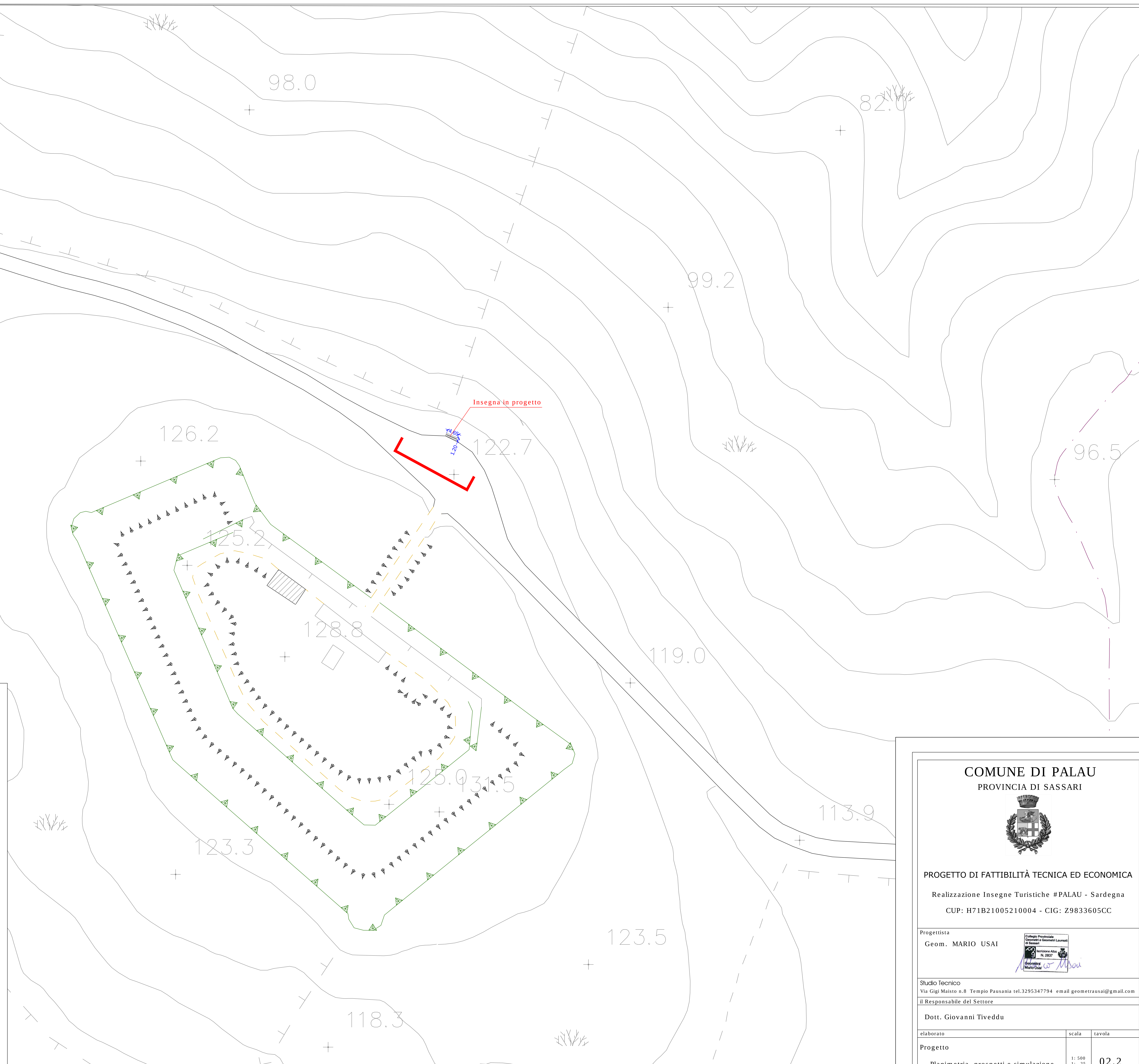
Planimetria opere in progetto scala 1:500
