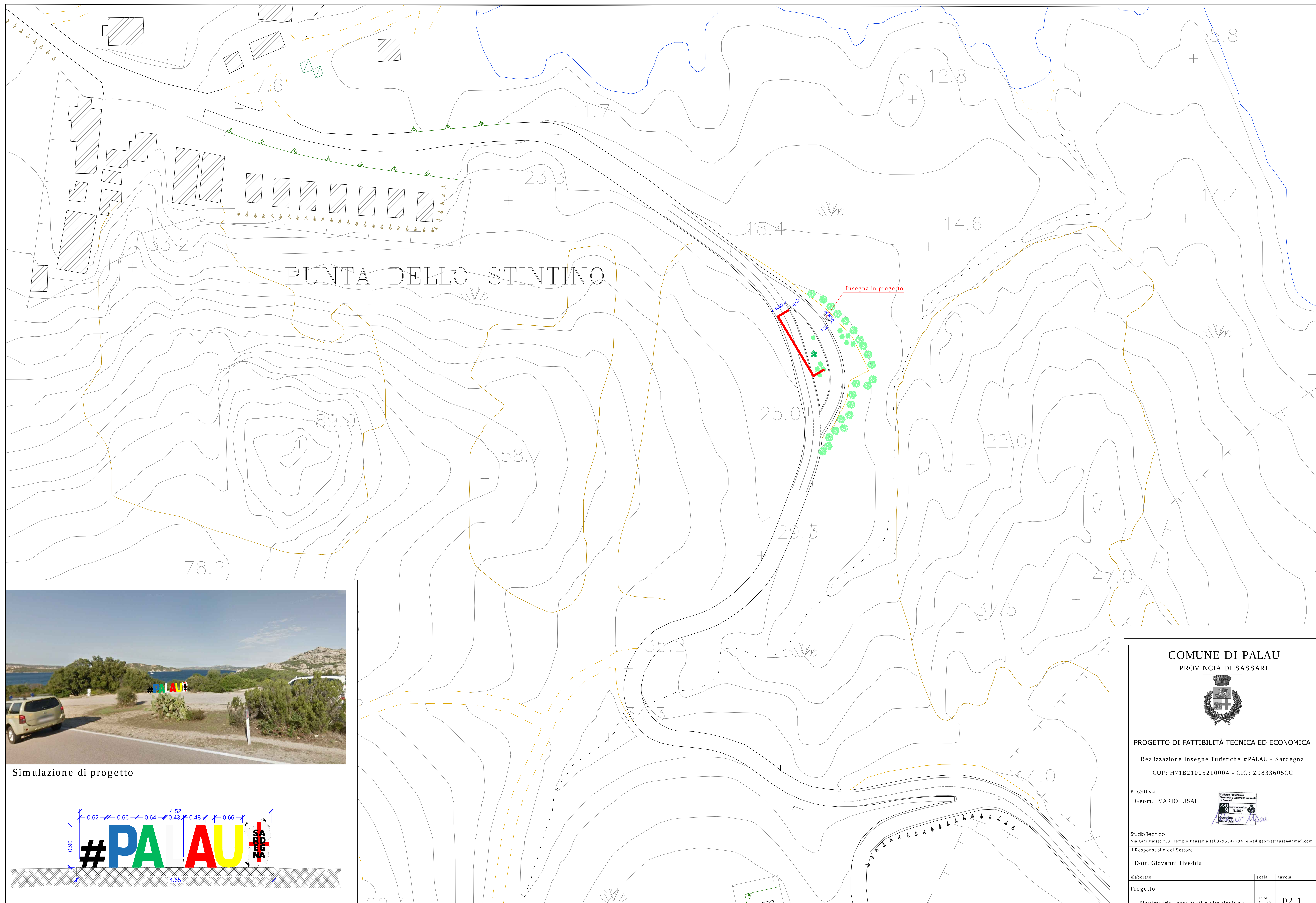
Prospetto Insegna scala 1: 25 Planimetria opere in progetto scala 1:500
